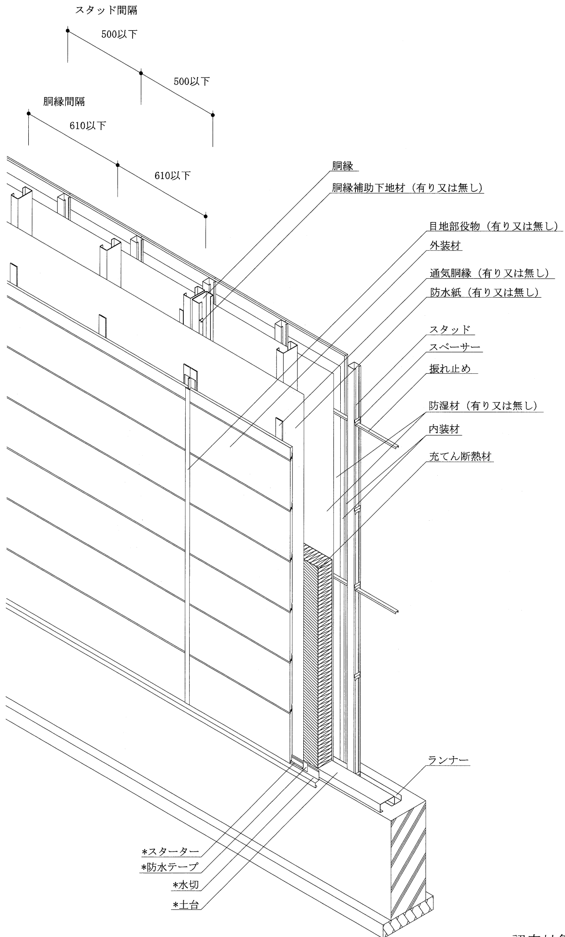
透視図 (別添-13)
